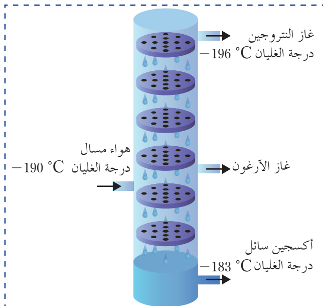
الشكل (2): التقطير الجزيئي للهواء المسال
