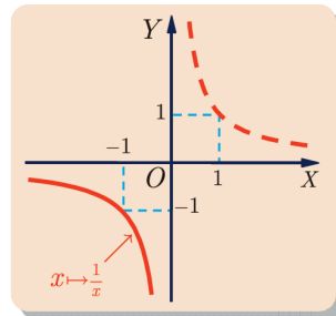
تابع المقلوب متناقصٌ تماماً على المجال ]-\infty, 0[
