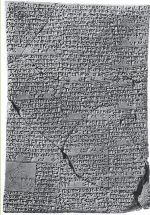
رقم بابلي قديم مكتوب بالمسمارية بحوي ست عشرة مسألة يؤول حل كل منها إلى معادلة من الدرجة الثانية
